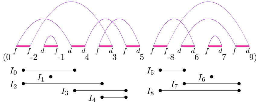
FIGURE 1.5 – Correspondance entre le graphe des breakpoints [52] et les intervalles élémentaires [10] pour la permutation P=(0-2-1 4 3 5-8 6 7 9) . Au-dessus de P est représenté le graphe des breakpoints avec ses arêtes du désir en traits fins et violets et ses arêtes de la réalité en traits épais et roses. Au-dessous, les 9 intervalles élémentaires, on remarque que ces intervalles et les arêtes du désir se correspondent.
